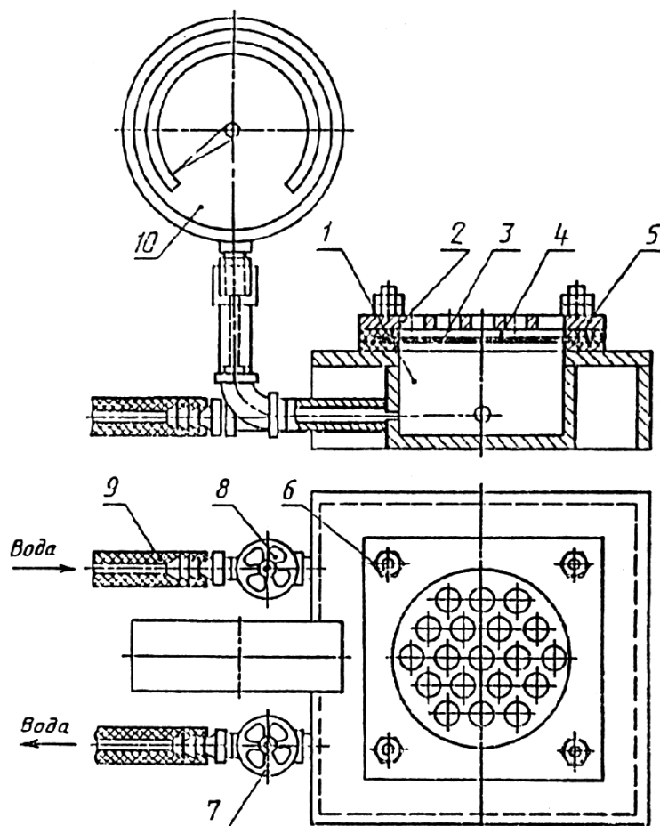
1 - рабочая камера; 2 - резиновые прокладки; 3 - образец; 4 - контактная сетка; 5 - прижимная плата; 6 - зажимные винты; 7, 8 - краны; 9 - резиновая трубка, соединяющаяся с водопроводом; 10 - манометр
