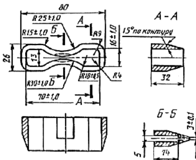
Рисунок Д.1 - Форма и угол заточки режущей кромки ножа для вырубki образцов-лопаток типа 1
