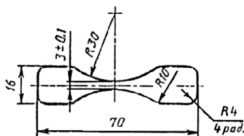
Рисунок 2 - Образец-лопатка типа 2
