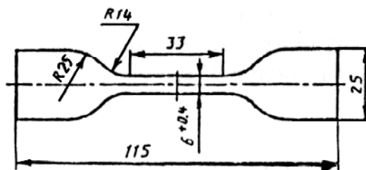
Рисунок 1 - Образец-лопатка типа 1
